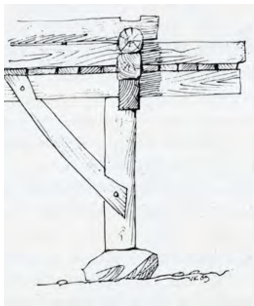
Dimenzije in prikaz povezave lesenega stebra na kamnitem podstavku z nosilnimi tramovi, ki povezujejo stebre v enovito podložno nosilno konstrukcijo nadgradnji – stenskemu ovoju in strehi. (Vir: Delavnica FA in TNP; Cevc, 1984, str. 59)
