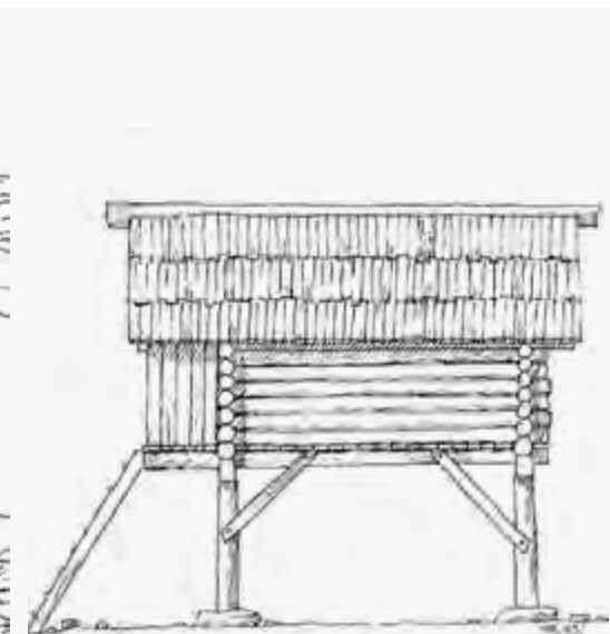
Lesen stan je postavljen na lesen podstavek, ki ga sestavlja štiri in več kobil. (Vir: Cevc, 1992, str. 79 in Cevc, 1984, str. 57)
