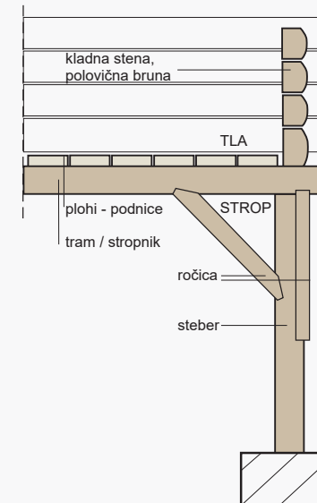
Prezrez stanu z vidno konstrukcijo lesene talne plošče, izdelane iz plohi, položenih na tramove – konstrukcijsko sestavino lesenega podnožja. (vir: Urh, 2005, str. 75) Planina Krstenica
