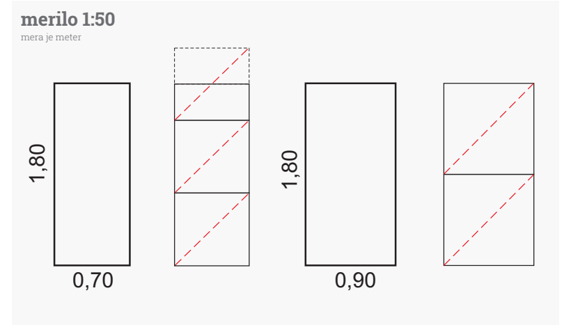
Skica najbolj pogostih dimenzij vratnih odprtin in razmerij med širino in višino vrat. Ti sta 1 : 2,5 (levo) in 1 : 2 (desno).
