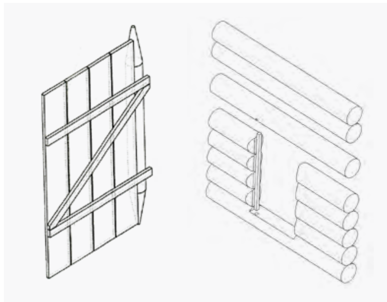
Shematski prikaz stavbnega pohištva, sestavljenega iz manjšega, pokončno postavljenega trama – »podloja«, lesenega tečaja ali »točaja« in vratnih kril. (Vir: Delavnica FA in TNP, Cevc, 1984, str. 108)
