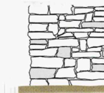
Stena iz grobo obdelanega ploščato lomljenega kamna; gradnja v plasteh, slojevita gradnja.
