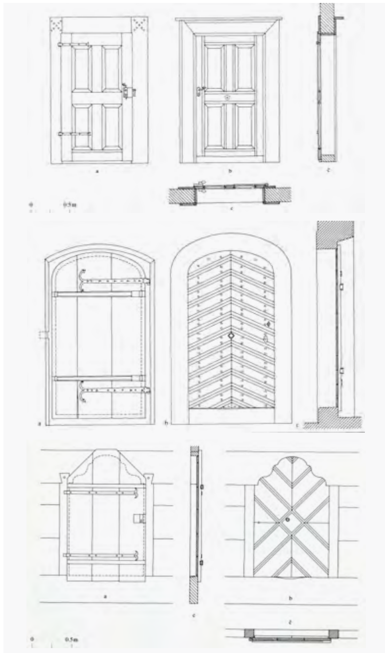
Konstruktivna skica prevladujoče oblike gladkih vratnih kril iz navpično položenih desk (zgoraj) in skice sočasno oblikovanih vrat v dolinskih naseljih (levo). (Vir: Cevc, 1984, str. 107 in Cevc, Primožič, 1991, str. 52, 53)
