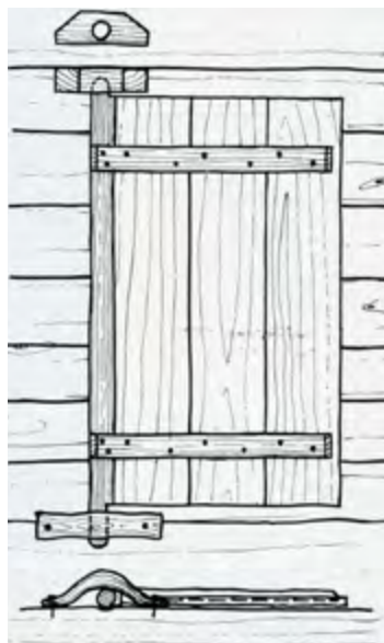
Shematski prikaz stavbnega pohištva, sestavljenega iz manjšega, pokončno postavljenega trama – »podloja«, lesenega tečaja ali »točaja« in vratnih kril. (Vir: Delavnica FA in TNP, Cevc, 1984, str. 108)
