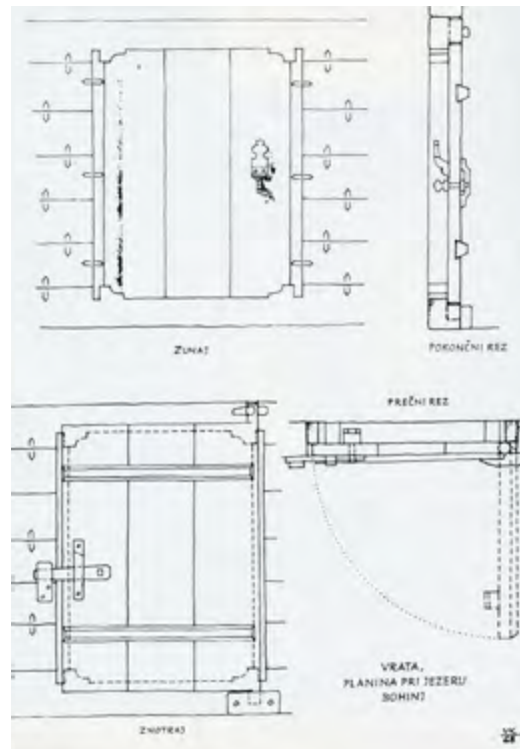
Konstruktivna skica prevladujoče oblike gladkih vratnih kril iz navpično položenih desk (zgoraj) in skice sočasno oblikovanih vrat v dolinskih naseljih (levo). (Vir: Cevc, 1984, str. 107 in Cevc, Primožič, 1991, str. 52, 53)
